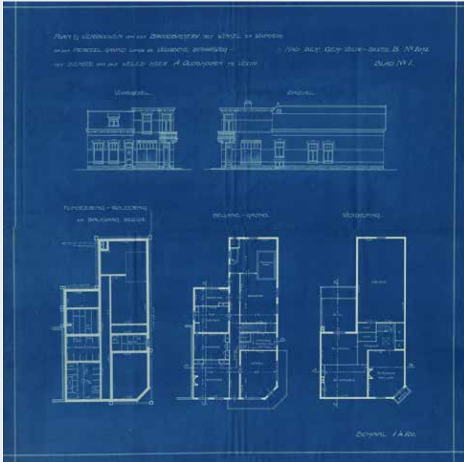
Originele blauwdruk behorende bij de aanvraag tot de bouw in 1919 Bron: bouwarchief gemeente Veur.
