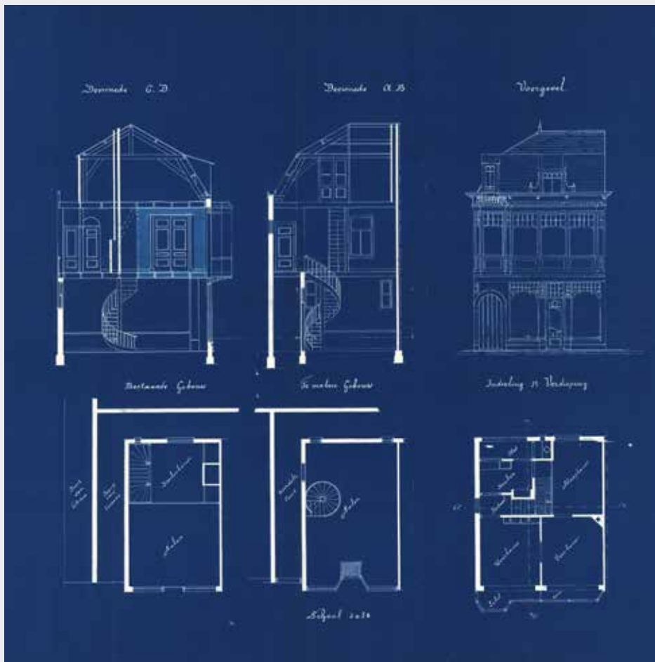
Originele bouwtekening van het pand Sluiskant 20 Bron: Bouwarchief Gemeentearchief Leidschendam-Voorburg.
