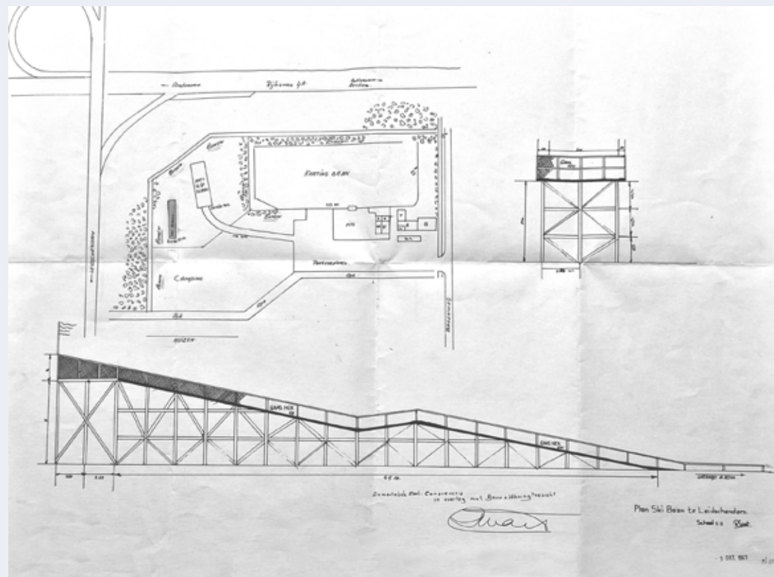
Plannen voor de realisatie van de skibaan in oktober 1963. Bron: Gemeentearchief Leidschendam-Voorburg.
