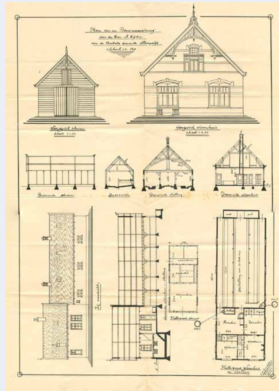
Schetsontwerp van de te realiseren bouwmanwoning aan de Broekweg, behorende bij de aanvraag van 3 juni 1911. Bron: Gemeentearchief Leidschendam-Voorburg.
