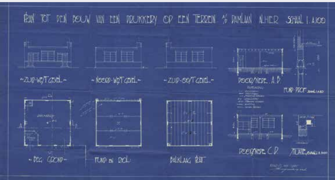
Blauwdruk van de te realiseren drukkerij aan de Damlaan van mei 1925 Bron: Bouwarchief Gemeentearchief Leidschendam-Voorburg
