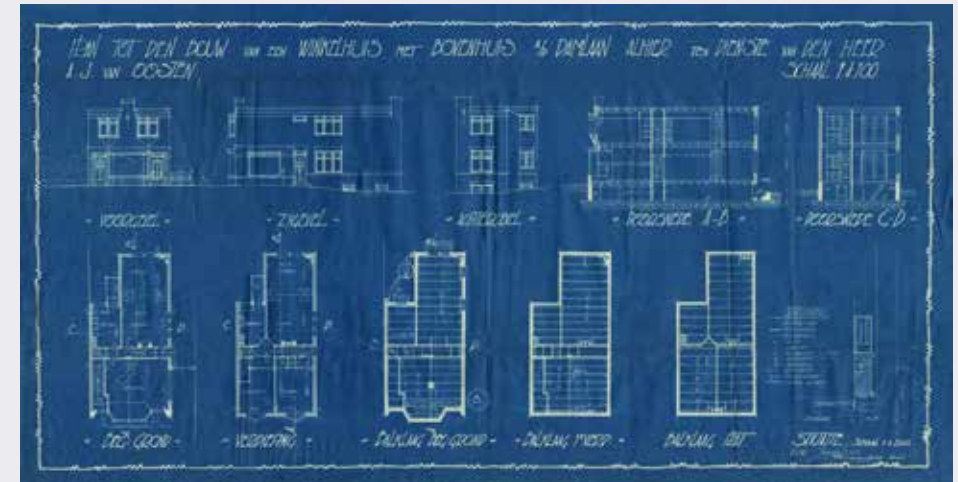
Originele blauwdruk van de bouw van een winkelhuis met bovenwoning aan de Damlaan. Bron: Gemeentearchief Leidschendam-Voorburg/ bouwarchief Leidschendam
