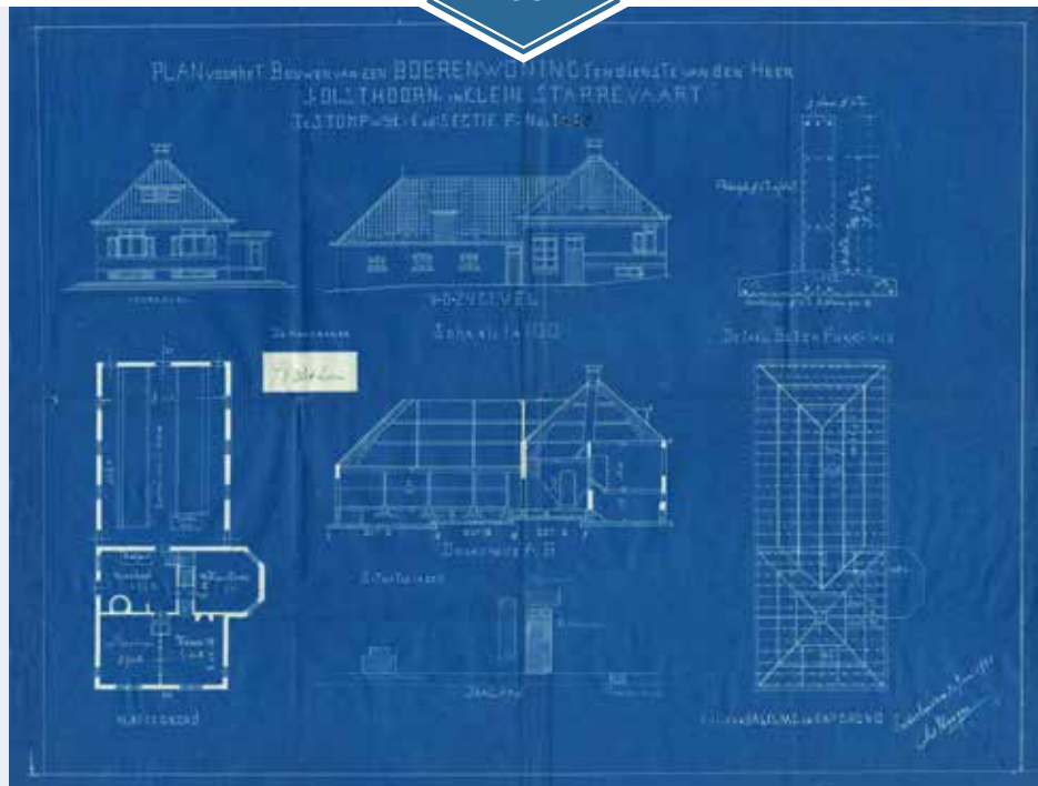
De originele bouwtekening bij de aanvraag voor het bouwen van een boerenwoning in opdracht van Johannes Jacobus Olsthoorn op 20 juni 1925. (Bron: Bouwarchief gemeentearchief Leidschendam-Voorburg)
